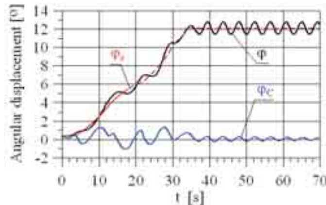
Fig. 8. Leveling error
